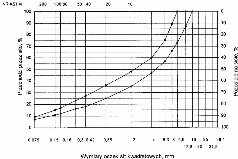
Rys. 7. Krzywe graniczne uziarnienia mieszanki mineralnej BA od 0 do 12,8 mm do warstwy ścieralnej nawierzchni
