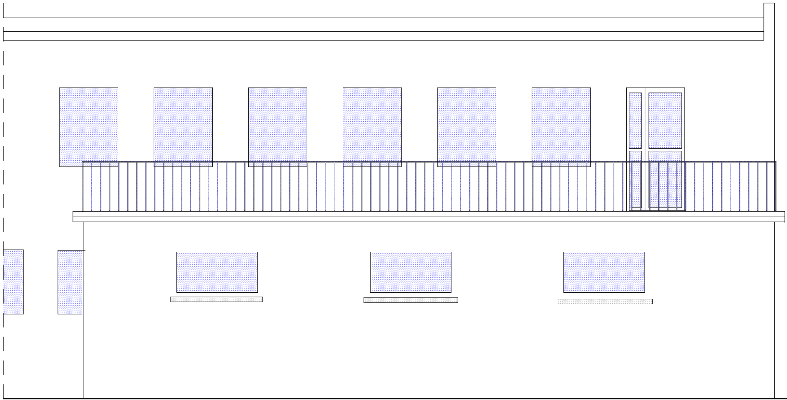
ELEWACJA POŁUDNIOWA
