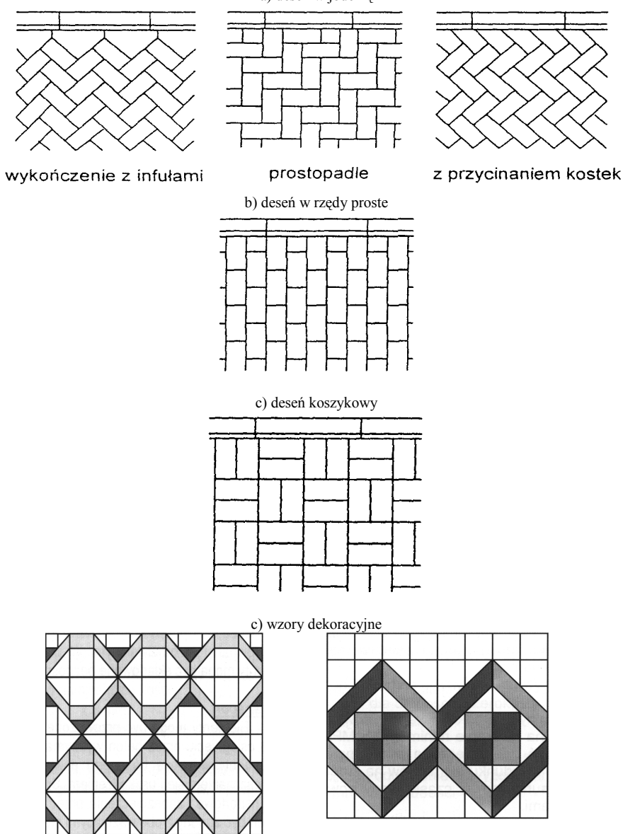
Załącznik 3. Przykłady deseni układania betonowych kostek brukowych (wg literatury podanej w zał. 1)
